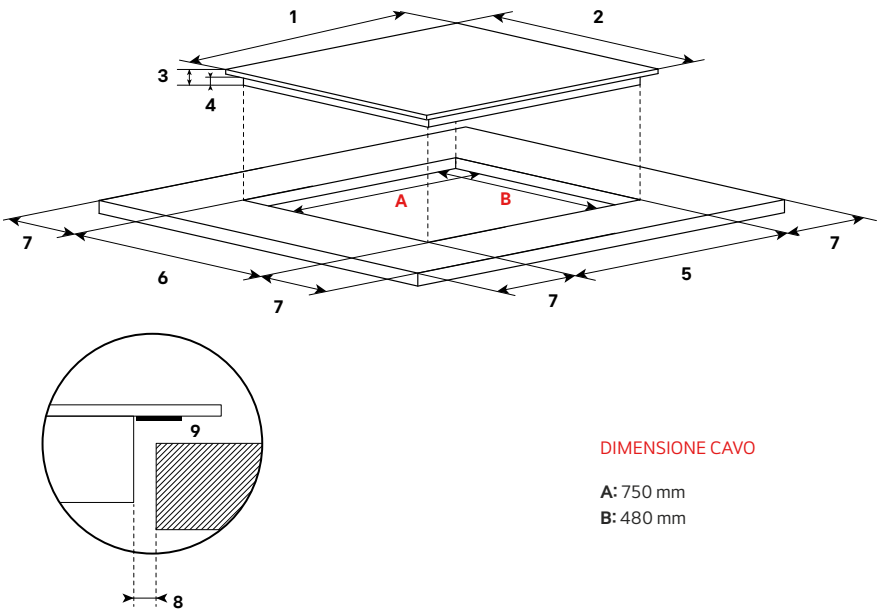
MISURE PER L'INSTALLAZIONE
