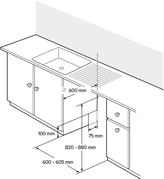
MISURE PER L'INSTALLAZIONE
