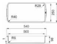
Vassoio contenitore
