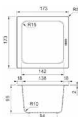
Vaschetta piccola
