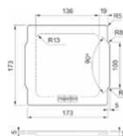
Coperchio legno
